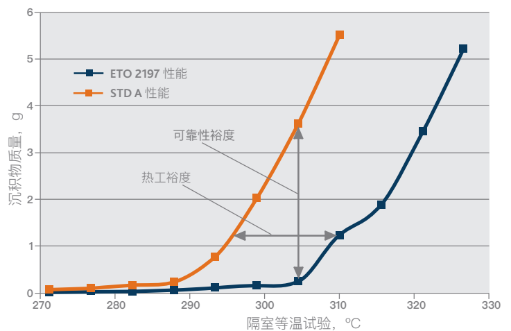
图1.ALADS将STD A 标准油的临界点与ETO 2197临界点比较
