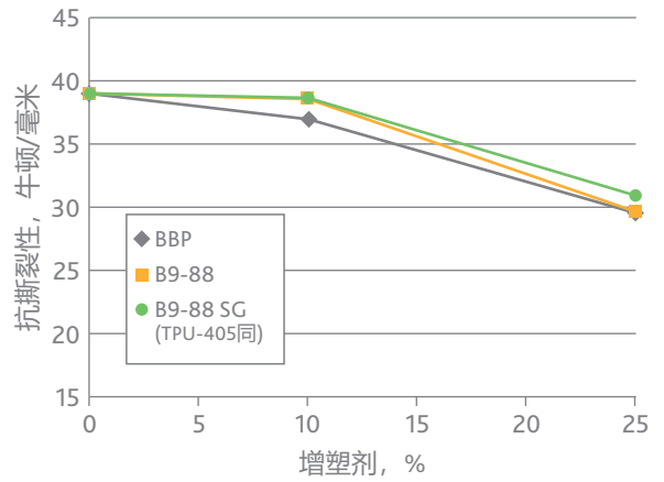
图5. MDI/聚酯TPU的抗撕裂性
