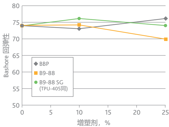
图3. MDI/聚醚基TPU的Bashore回弹性
