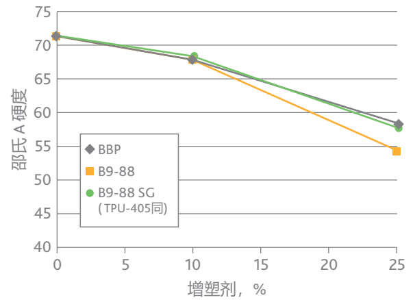
图4. MDI/聚酯TPU的邵氏A硬度
