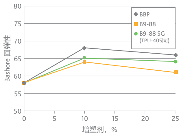
图6. MDI/聚酯TPU的Bashore回弹性
