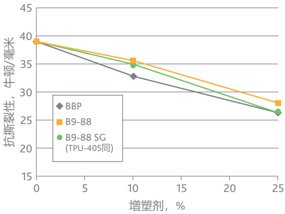
图2. MDI/聚醚基TPU的抗撕裂性
