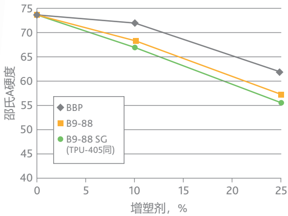
图1. MDI/聚醚基TPU的邵氏A硬度
