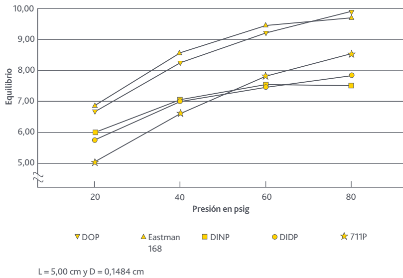
Figura 4 Viscosidad Severs, 48 horas de añejamiento
