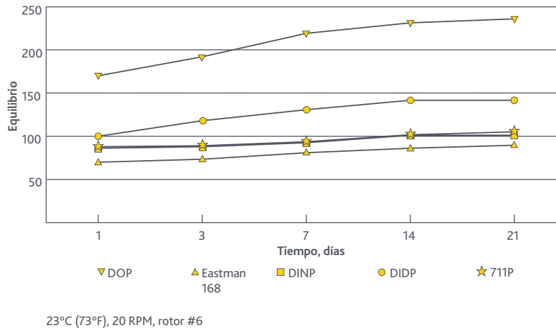
Figura 3 Viscosidad Brookfield
