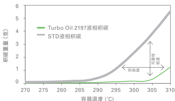
液相积碳: Eastman Turbo Oil 2197与STD相比
