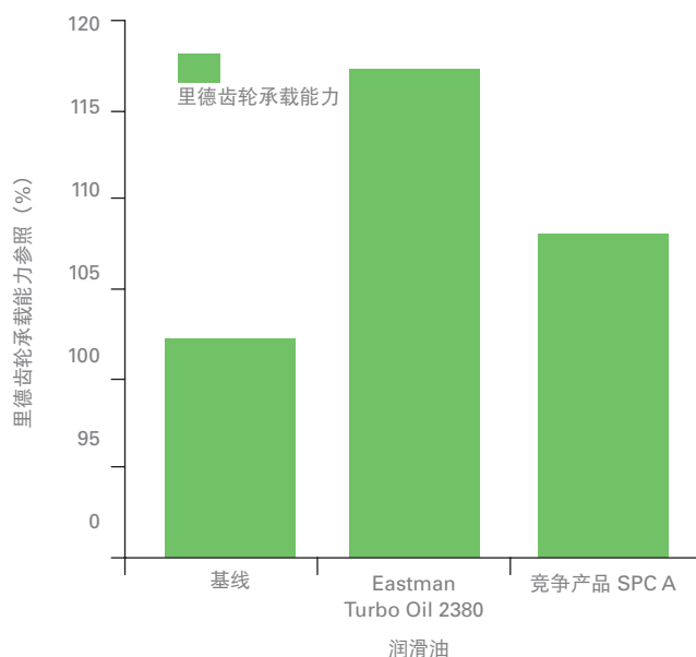
里德齿轮承载能力
