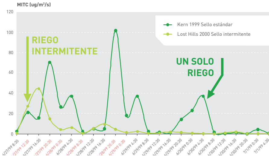
Comparación de flujo de MITC a la atmósfera durante un período de control de 96 horas con 24 muestreos a intervalos de 4 horas entre campos tratados con metam bajo riego intermitente y un solo riego.
