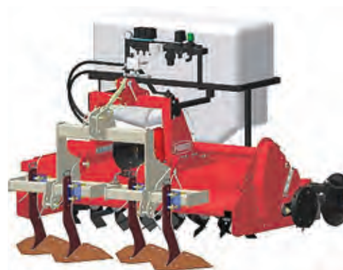
Rotativa con inyección (fabricada por Imants)
