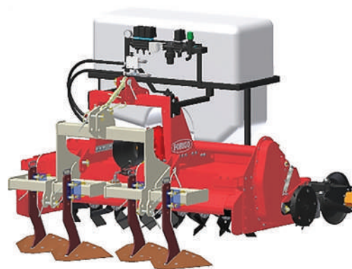
● Macchina di disinfezione del terreno Mix Tiller Deeper (prodotta da FORIGO)
