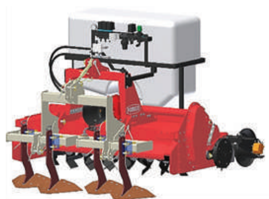
● Máquina para desinfección de suelos con cultivador de mezcla más profunda (fabricada por Forigo)
