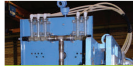
Medidor de flujo de varios canales
