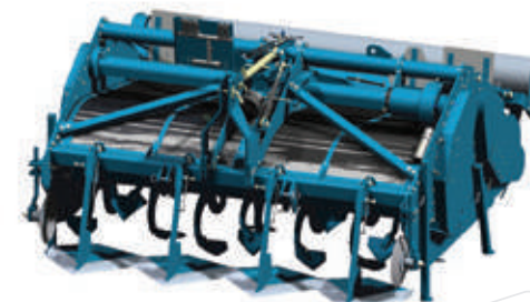
● Rotativa con inyección (fabricada por Imants)
